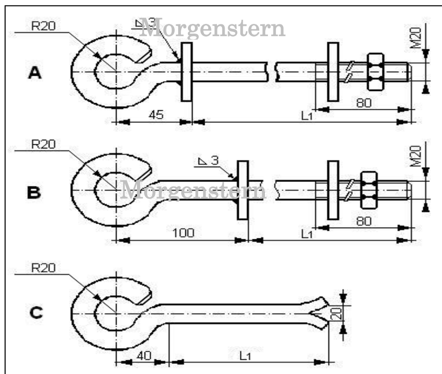
Abspannöse für Luftkabel Typ NF 2AX Form A, B, C mit gebogener Öse
