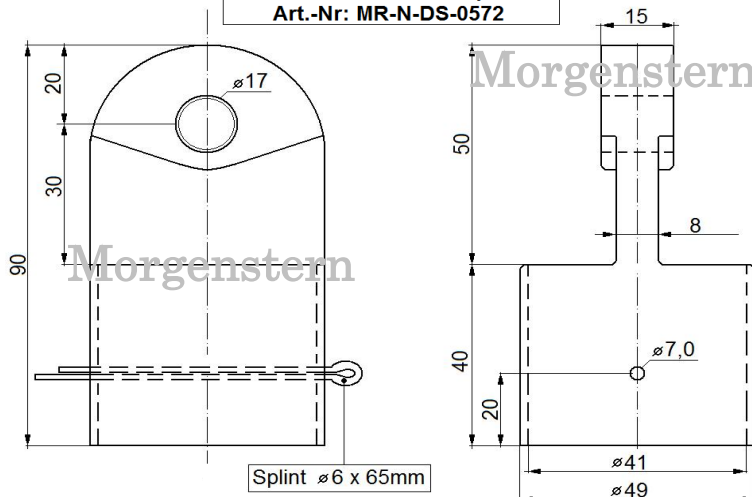
T-Anschlusslasche / Kopfstück Art.-Nr: MR-N-DS-0572
